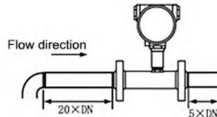
90° bend
